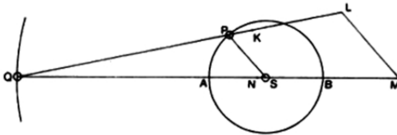
Figura 8. El diagrama ha sido reconstruido a partir del texto, por analogía con el diagrama de la proposición LXVI. El diagrama original no ha sobrevivido.
