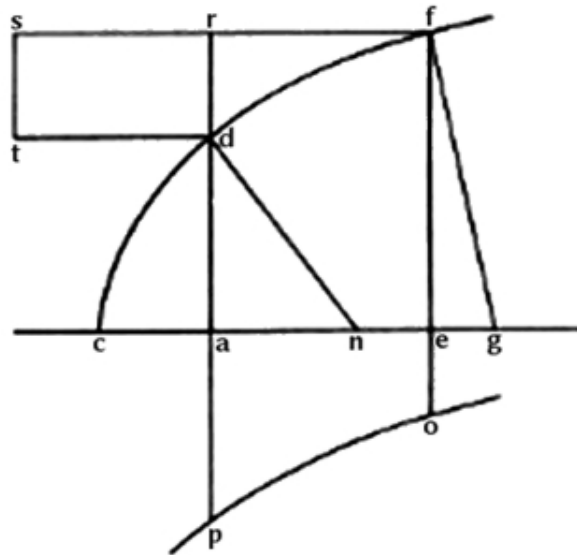
Figura 1. Teorema fundamental del cálculo
