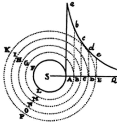
Figura 9. La dinámica de un vórtice.
