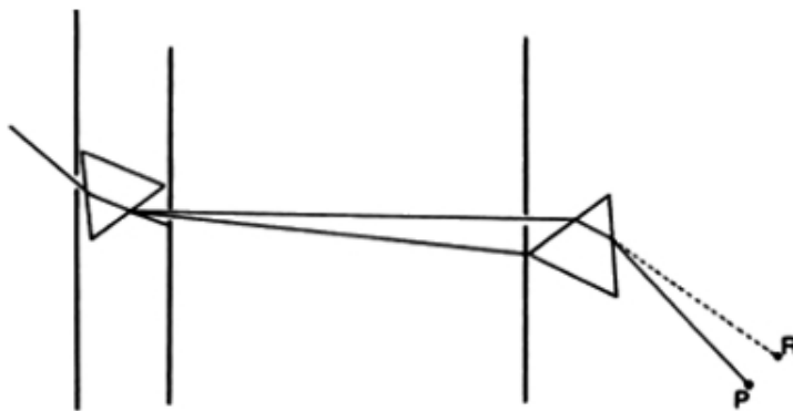
Figura 4. El experimentum crucis .
