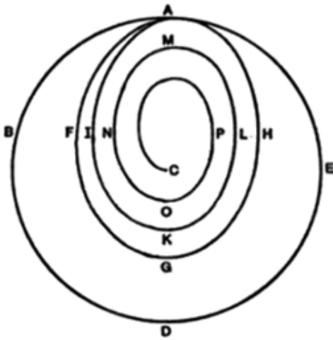
Figura 7. AFGH es la trayectoria elíptica de un cuerpo que no encuentra ninguna resistencia. La espiral interior AIKLMNOPC representa su camino en un medio resistente.
