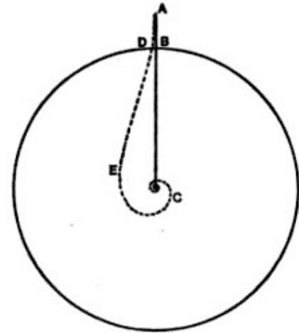
Figura 6. Dibujo de Newton sobre el camino recorrido por un cuerpo que cae sobre una tierra en rotación.
