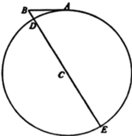
Figura 3. La fuerza de un cuerpo moviéndose en un círculo derivada de su desviación de la tangente
