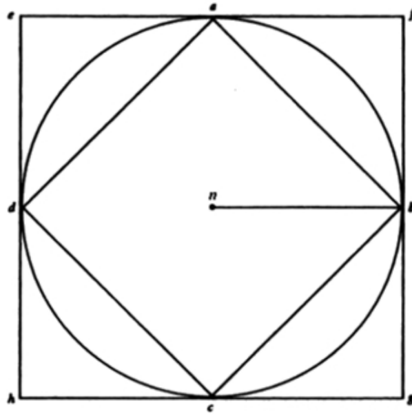
Figura 2. La fuerza de un cuerpo moviéndose en un círculo derivada de un impacto.
