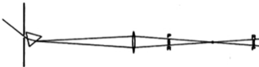
Figura 5. La reconstitución de la luz blanca con una lente.
